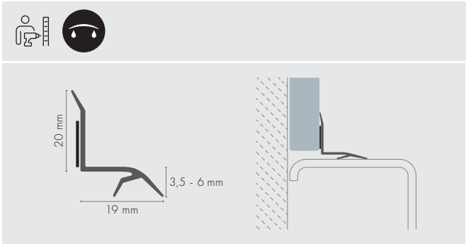
PROFIL WANNOWY SAMOPRZYLEPNY SELF-ADHESIVE BATHTUB PROFILE SELBSTKLEBENDES WANNENPROFIL
