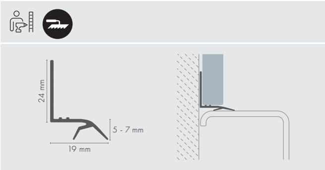
PROFIL WANNOWY PODPŁYTKOWY UNDER-TILE BATHTUB PROFILE UNTERFLIES-WANNENPROFIL
