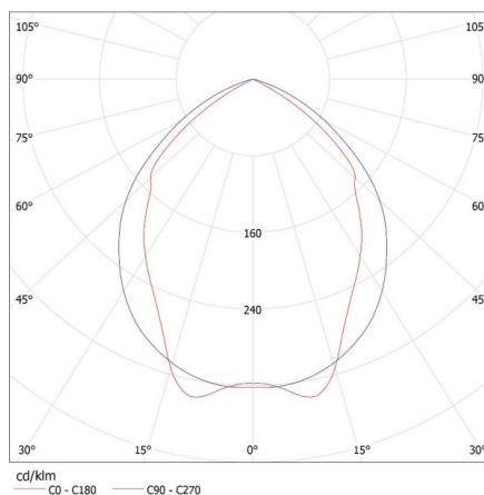
KANLUX S.A. (kat 22671) NOTUS 4LED 418 NT + GLASSv2 / Krzywa rozsyłu światła (biegunowo)
