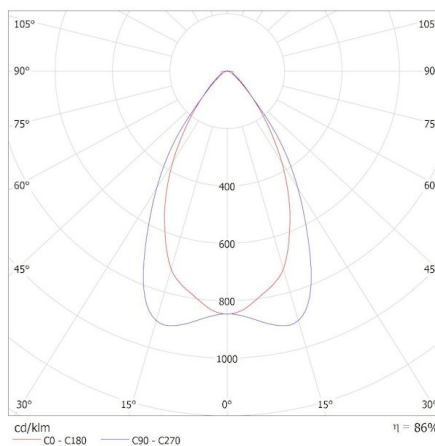
KANLUX S.A. (kat 37543) KNU-L6D-WW-B-P1D / Krzywa rozsyłu światła (biegunowo)
