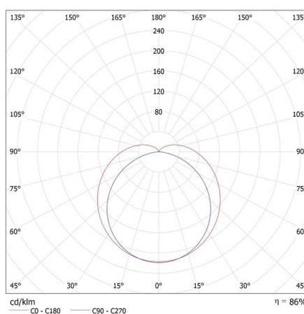
KANLUX S.A. (kat 38941) TP SLIM N 50W-NW / Krzywa rozsyłu światła (biegunowo)
