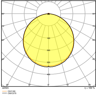
PL CMFT 600 P 33W 830 PS
