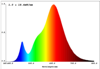
VALEDIS60 7W 840 GLFR
