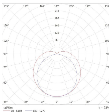
KANLUX S.A. (kat 38940) TP SLIM N 40W-NW / Krzywa rozsyłu światła (biegunowo)
