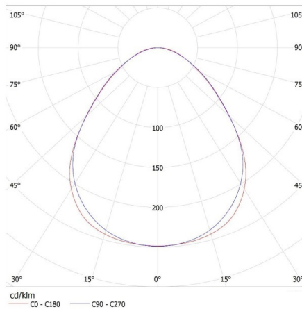
KANLUX S.A. (kat 28445) AL 4LED 60-MPR-SR + GLASSv2 / LDC (Polar)
