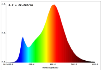
VALEDIS100 11W 827
