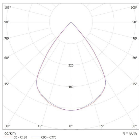
KANLUX S.A. (kat 34102) AL-LL-WW-RST-B-NT / Krzywa rozsyłu światła (biegunowo)
