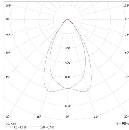
KANLUX S.A. (kat 37536) KNU-S6D-WW-W-P1D / Krzywa rozsyłu światła (biegunowo)
