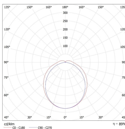
KANLUX S.A. (kat 33163) TP STRONG 60W 12 NW / Krzywa rozsyłu światła (biegunowo)
