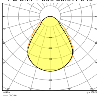
PL CMFT 600 29.5W 930
