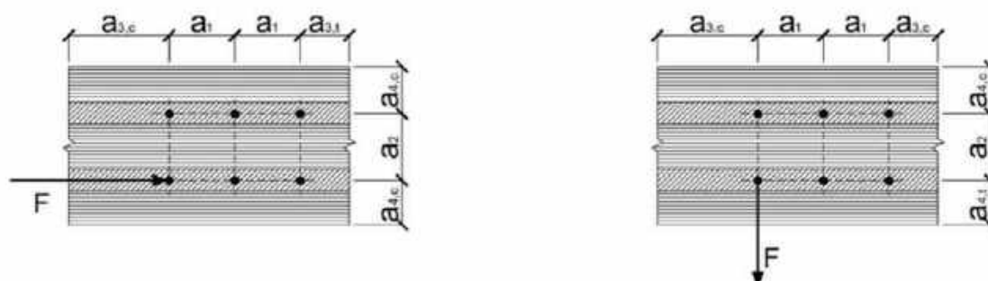
Rys. A.2.2 Definicja odstępów, odległości między końcami i krawędziami na powierzchni bocznej drewna klejonego krzyżowo. W przypadku wkrętów w powierzchni bocznej a1 i a3 są równoległe do powierzchni płaskiej CLT, a a2 i a4 prostopadłe do powierzchni płaskiej.
